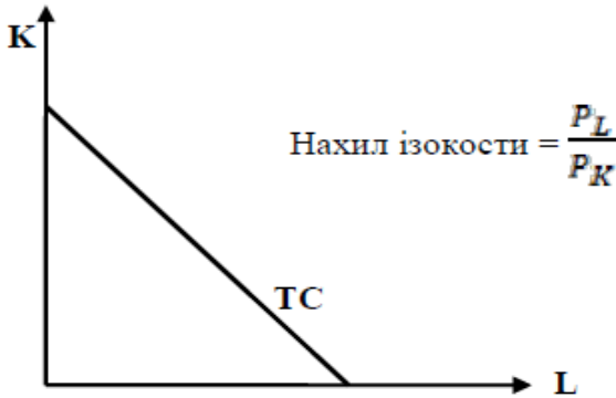
Рис. 6.3. Ізокоста
