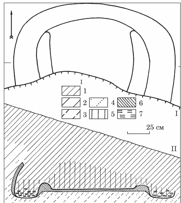
Рис. 1. Гончарний горн з Чернівців: I — план; II — профіль; умовні позначки: 1 — чорний суглинок; 2 — жовто-сірий суглинок; 3 — жовтий супісок; 4 — перепалений ґрунт; 5 — залягання кераміки; 6 — глиняна обмазка з домішкою органіки; 7 — попіл та вуглики
