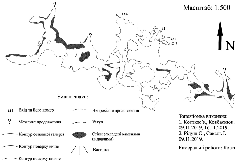
Рис. 18. Картошхема печери Вишневої
