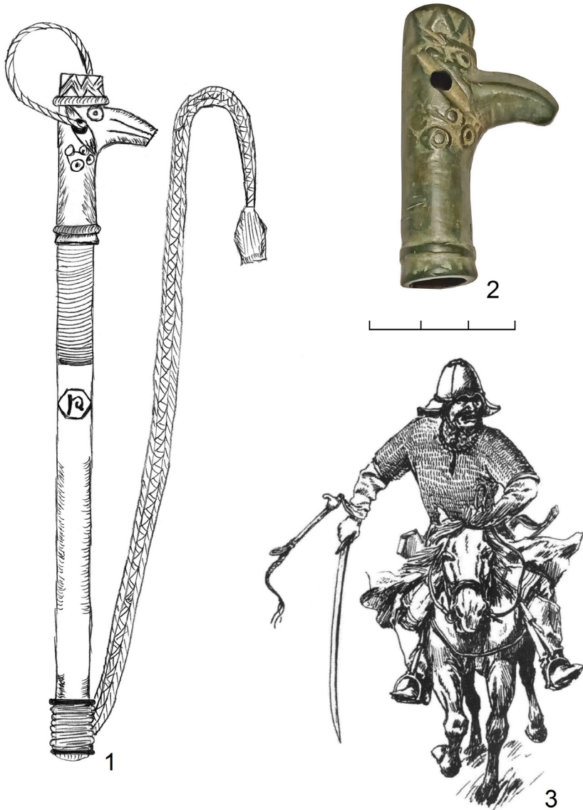
Рис. 1. 1 – реконструкція пліті, 2 – наверхя пліті з городища, 3 – використання пліті середньовічними кочівниками (за В.Н.Чхейдзе).
