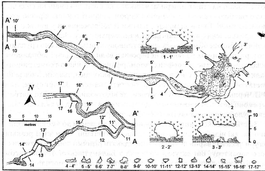
Рис. 1. Баламутівська печера. План та розрізи. (Топографічна зйомка Чернівецького спелеоклубу "Троглодит").
