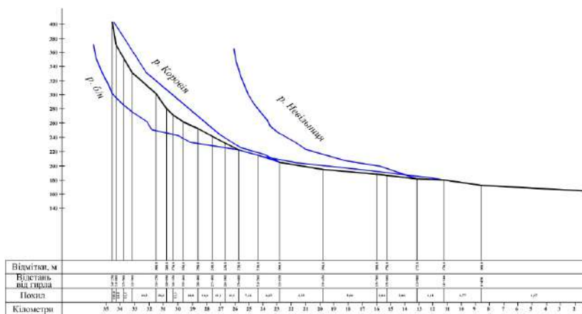
Рис. 2.32. Поздовжні профілі основних приток р. Дерелюї
