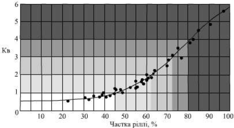
Рис. 2.40. Номограма розрахунку впливу ріллі на коефіцієнт відносної напруженості
