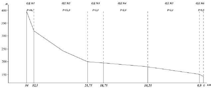
Рис. 2.22. Поздовжній профіль річки Дерелую з розбиттям його на однорідні ділянки
