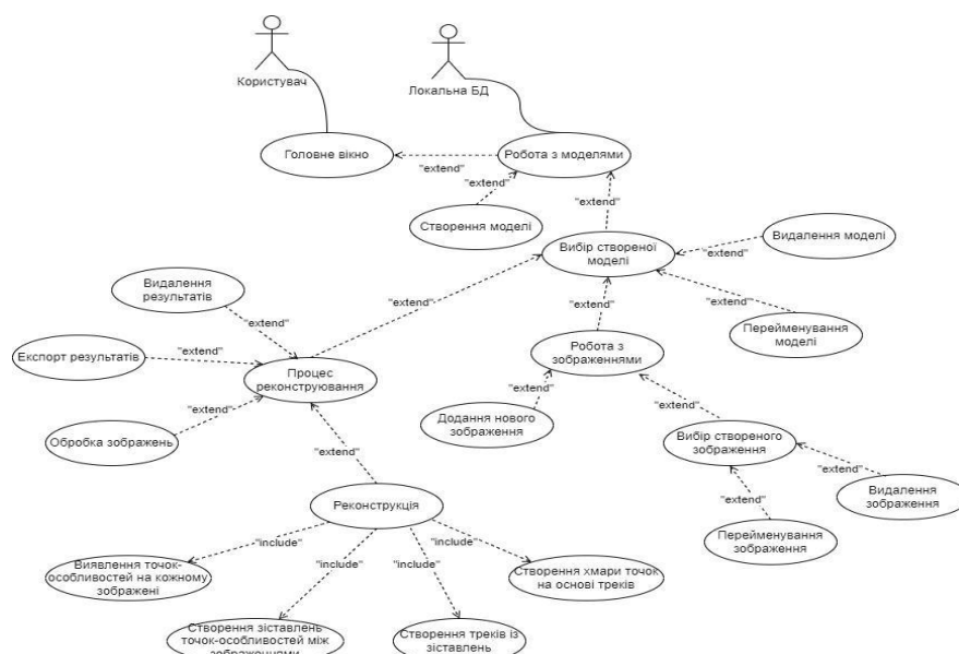
Рис. 1. Діаграма варіантів використання інформаційної системи
