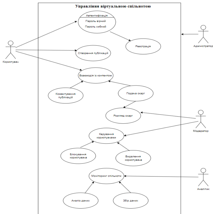
Рис. 4. UML-діаграма прецедентів
