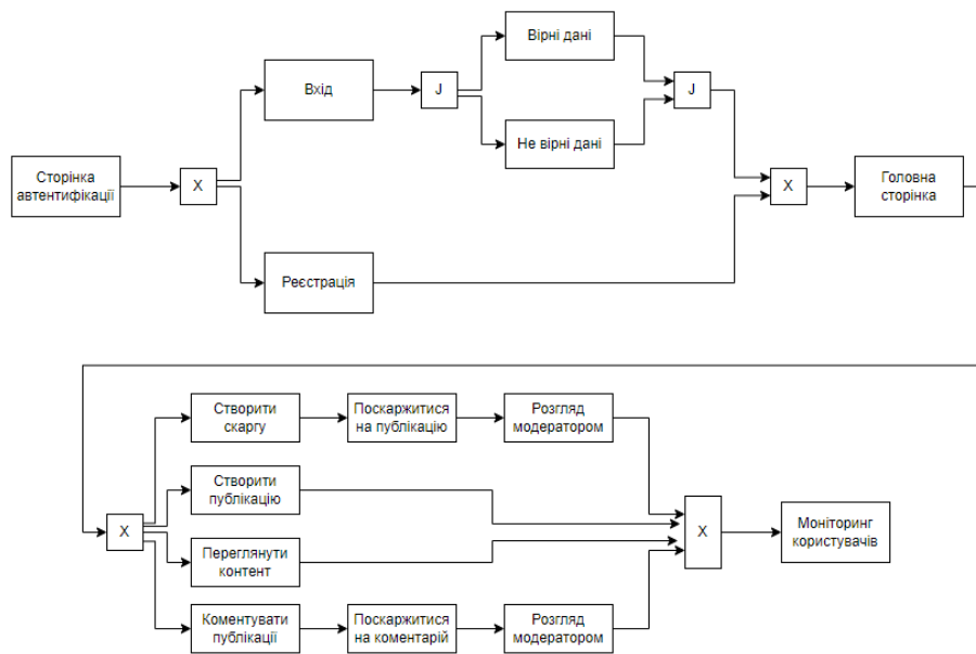
Рис. 3. IDEF-3 діаграма
