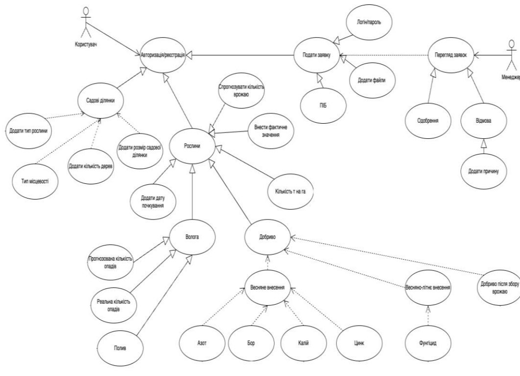
Рис. 1. Діаграма варіантів використання системи
