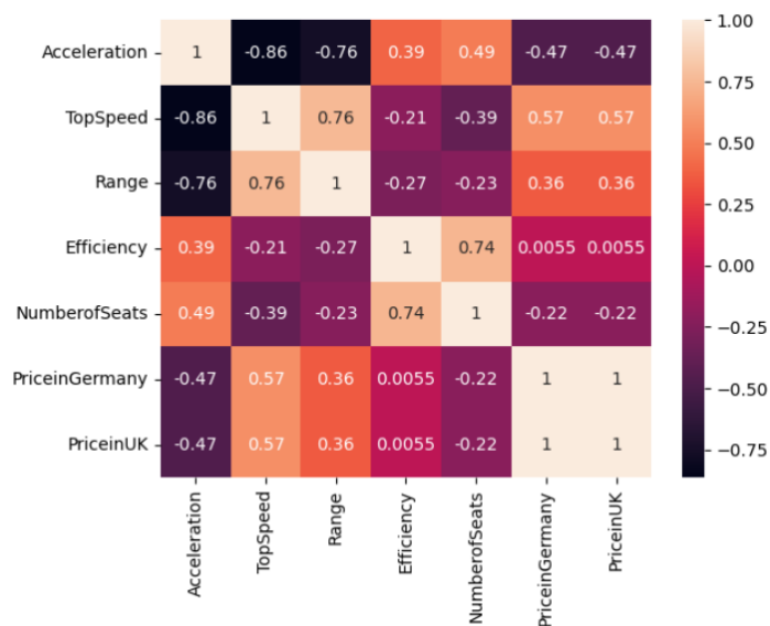
Рис. 3. Heatmap для кореляційної матриці
