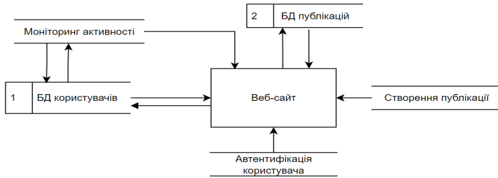
Рис. 1. DFD-діаграма
