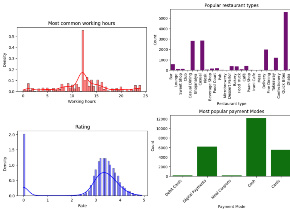
Рис. 1. Розподіл даних
