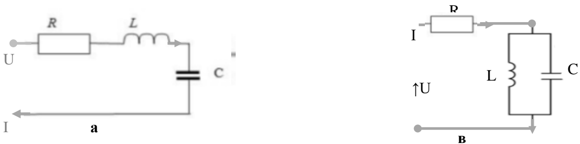
Рис. 2. Пара RLC схем за умов резонансу: а – струму, в – напруги.
