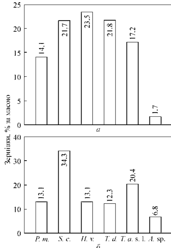
Рис. 2. Палеоетноботанічний спектр зернівок злакових культурних рослин за масою: а – Комарів; б – Глинське; P. m. – Panicum miliaceum (просо); S. c. – Secale cereale (жито); H. v. – Hordeum vulgare (ячмінь півчастий); T. d. – Triticum dicoccon (пшениця двозернянка); T. a. s. l. – Triticum aestivum s. l. (пшениці м'які голозерні); A. sp. – Avena sp. (овес).
