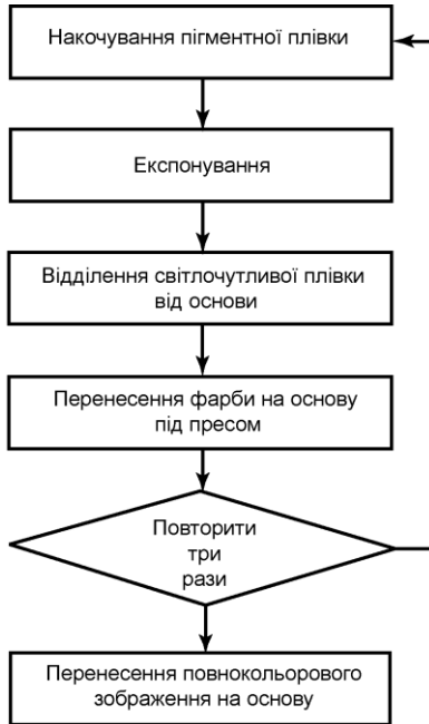
Рис. 27 Створення зображення за допомогою установки DuPont Cromalin Studio Sprint
