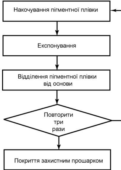
Рис. 25 Схема створення зображення за допомогою установки AGFA PressMatch Dry
