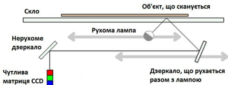
Рис.1 Принцип роботи планшетного сканера
