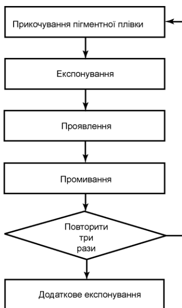
Рис. 24 Схема створення зображення за допомогою «мокрої» кольоропроби
