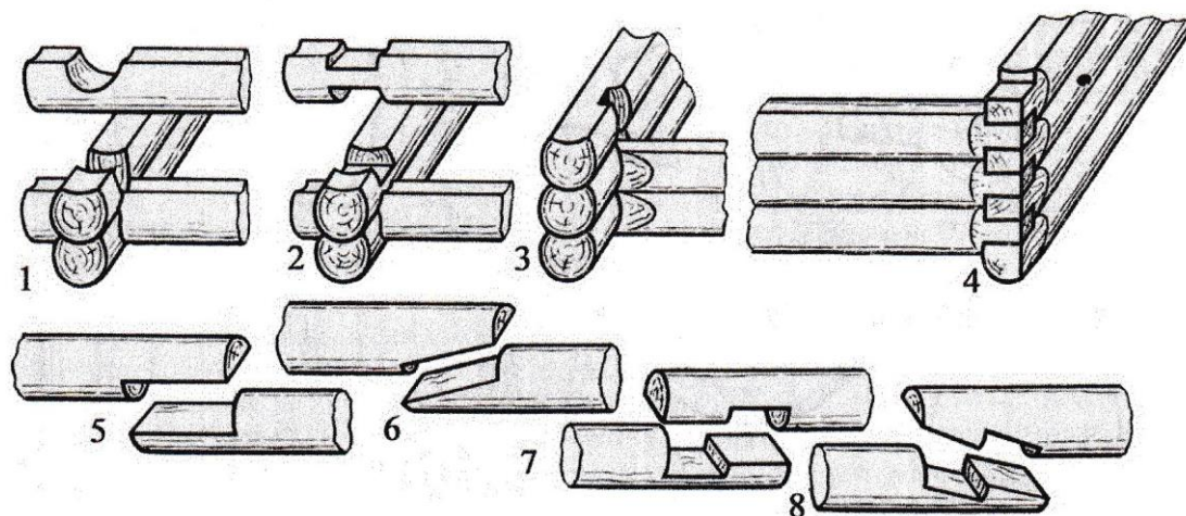
Рис. 5. Зразки дерев'яних з'єднань (за Б.О. Колчиним [1985, табл. 103])
